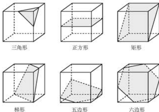
图 11 正方体截面图形示意图
